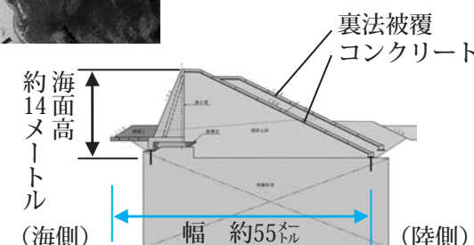
標準断面図（案）
