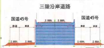
セパレート区間横断面図
