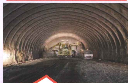
白井トンネル 掘削工
